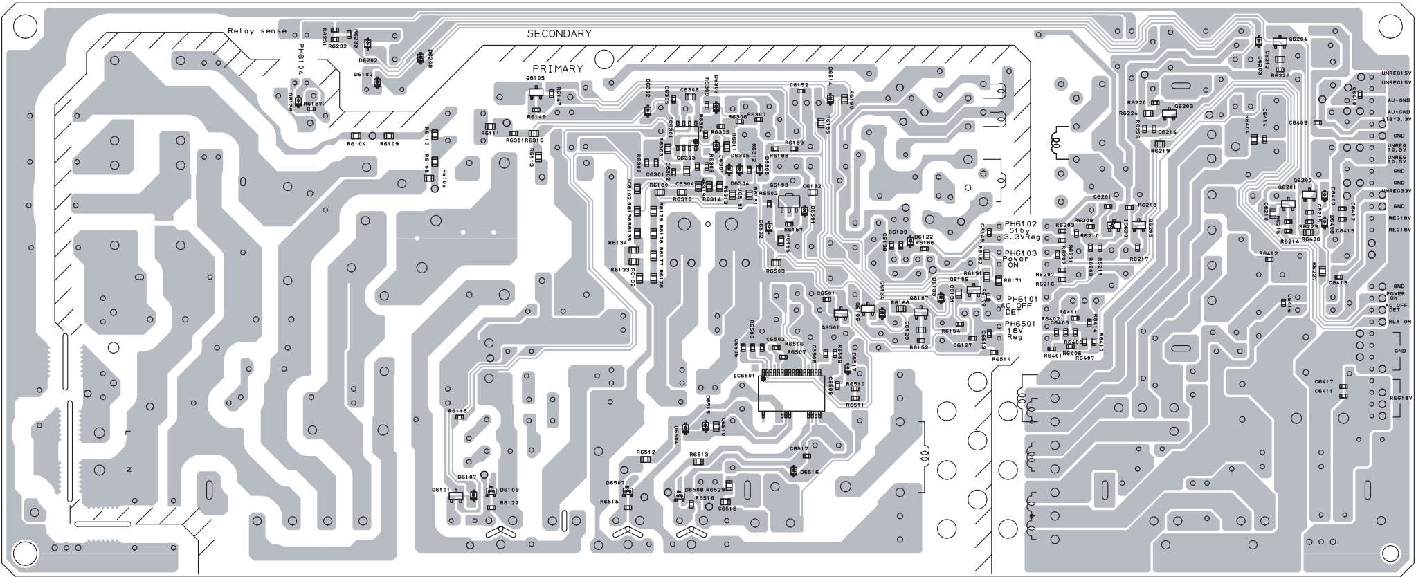
<CONDUCTOR SIDE>
