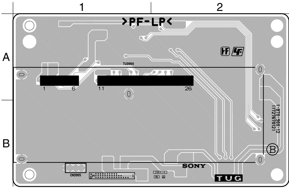
<CONDUCTOR SIDE>
